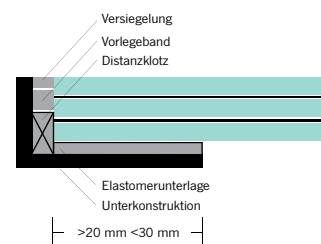
Linienförmige Lagerung einer begehbaren Verglasung
